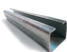
CP555 Válcovaný nosný „C“ profil 97(š) x 90(v) mm se stěnou o síle 5,5 mm pro samonosné brány bez povrchové úpravy. Viz str. 180
