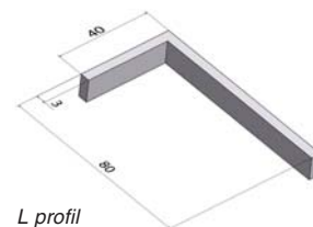
L profil
