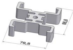
TKS profil
