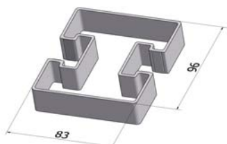
HP profil
