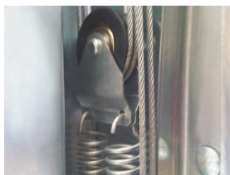
pružinový systém s kladkou
