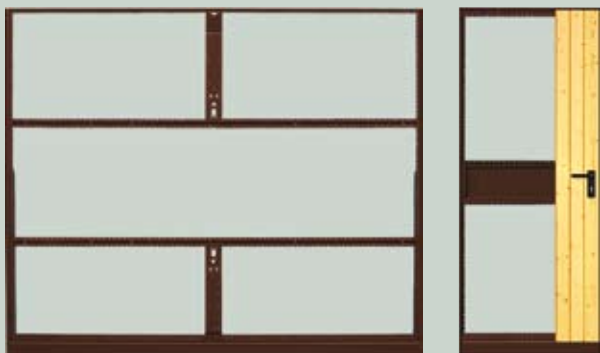
905 pro vlastní výplň stavebníka ●
