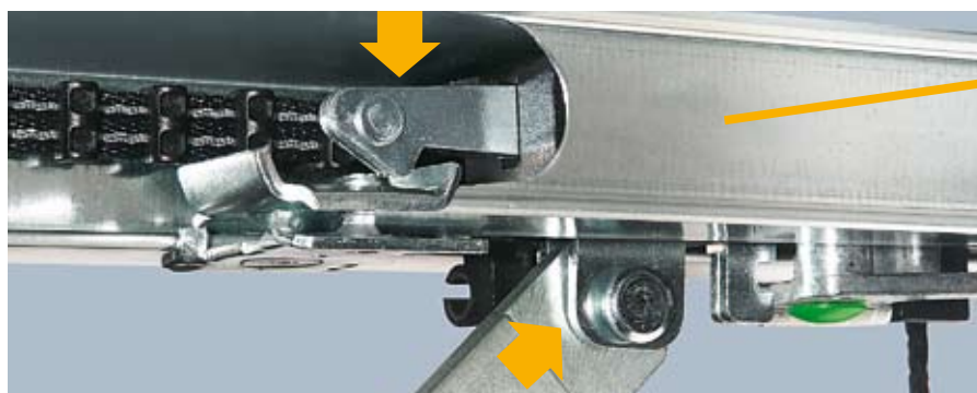
Uzavření vrat v kolejnici pohonu - patent společnosti Hörmann
