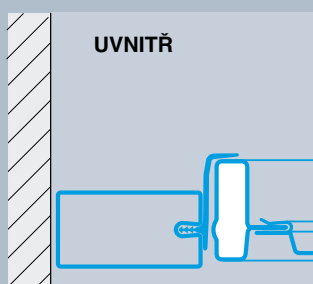
Typ vrat N80 Doraz v otvoru
