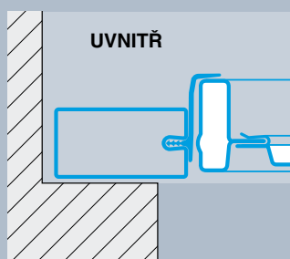
Typ vrat N80 Doraz za otvorem
