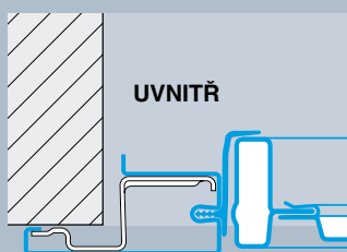
Typ vrat F80 Doraz před otvorem
