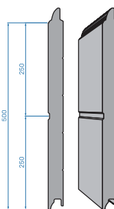
drážka
