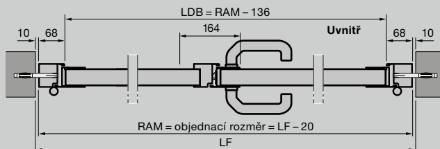
2křídlové vedlejší dveře s hliníkovou blokovou zárubní, typ profilu 2 Montáž v otvoru
